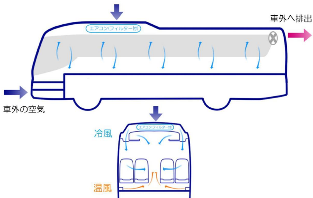
HINOセレガ・ISUZUガーラ 車内空調イメージ図
